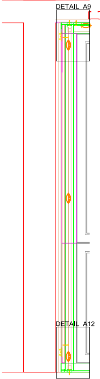
SECTION A2
